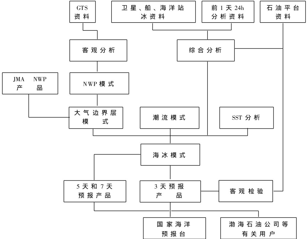
图 4 渤海海冰数值预报流程图
