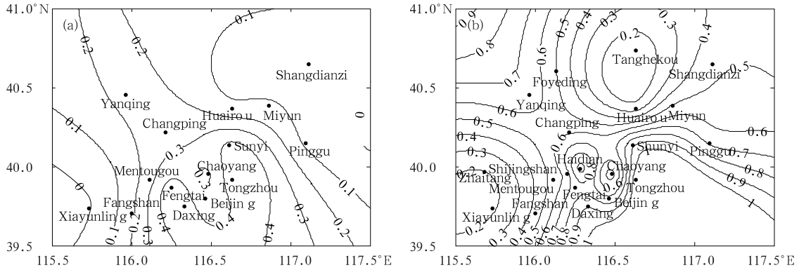
图2 北京地区年平均温度变化速率
