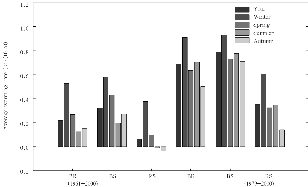
图1 1961~2000和1979~2000年北京地区国家基本/基准站(BR)、北京站(BS)和乡村站(RS)平均增温速率(单位: ^{\circ}\text{C}/(10\text{ a}) )
