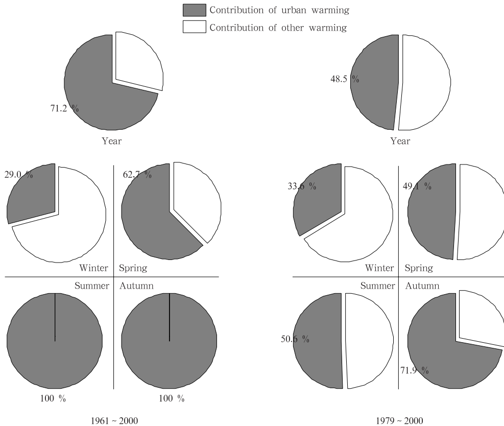
图3 1961~2000和1979~2000年北京地区国家基本/基准站(BR)热岛增温贡献率(%)
