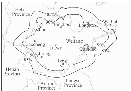
图 1 山东省电力雷电监测定位网分布情况 (圆圈表示雷电探头位置) Fig. 1 Locations of lightning detection network in Shandong Province
