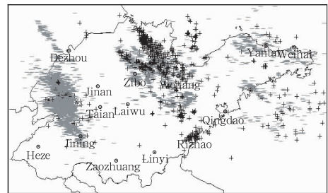
图 2 2002 年 6 月 1 日全天内山东地区地闪分布情况 (负地闪用“-”表示,正地闪用“+”表示) Fig. 2 Spatial distribution of total cloud-to-ground flashes on 1 June, 2002 (-: negative CG lightning; +: positive CG lightning)
