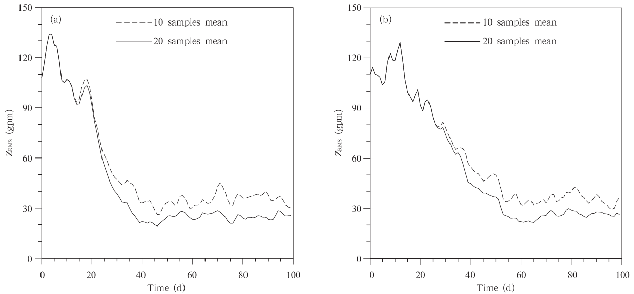
图 1 由 SAMIL 模拟得到的两组 REME 试验的 500 hPa 位势高度场结果之间的均方根误差随时间的变化 (第 1、2 组 REME 试验的初始场分别为第 30 年 1 月 1 日和第 31 年 1 月 1 日; a. 单精度试验结果, b. 双精度试验结果) Fig. 1 Temporal evolution of the RMS (unit: gpm) of 500 hPa geopotential height between two SAMIL REME experiments under the computational mode of (a) single precision and (b) double precision and with initial conditions taken from those on the 1st day of the 30th and 31st integration year of a 60 years stable climate simulation (control run)
