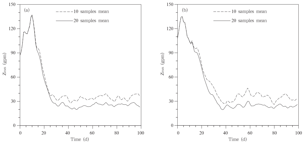
图 2 由 SAMIL 模拟得到的两组 REME 试验 500 hPa 位势高度场结果之间的均方根误差随时间的变化 (第 1、2 组 REME 试验的初始场分别为第 30 年 6 月 1 日和第 31 年 6 月 1 日; a. 积分时间步长为 900 s, b. 积分时间步长为 600 s) Fig. 2 Temporal evolution of the RMS (unit: gpm) of 500 hPa geopotential height between two SAMIL REME experiments under a time step of (a) 900 s (b) 600 s, and with initial conditions taken from those on the 1st day of June of the 30th and 31st integration year of a 60 years stable climate simulation (control run)
