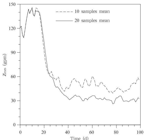
图4 由ECHAM5模拟得到的两组REME试验500 hPa位势高度场结果之间的均方根误差随时间的变化(第1、2组REME试验的初始场分别为第30年1月1日和第31年1月1日;虚线是每组REME试验选取10个样本得到的结果,实线同虚线但REME试验样本数为20)
