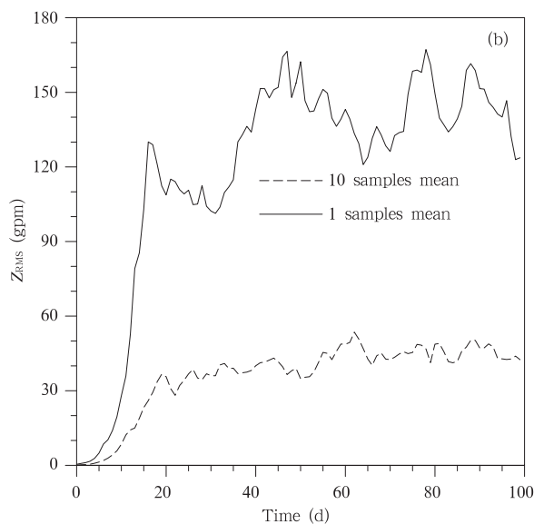
图5 由ECHAM5模拟得到的两组REME试验500 hPa位势高度场结果之间的均方根误差随时间的变化 (a. 虚线是每个初始场选10个样本做REME得到的结果,第1、2组REME试验的初始场分别为第30年1月1日和第31年1月1日,实线是第30年1月1日的试验前10个样本REME试验和后10个样本REME试验结果之间的RMS差别; b. 虚线是第30年1月1日的试验前10个样本REME试验和后10个样本REME试验结果之间的RMS差别,实线同虚线,但样本个数为1)
