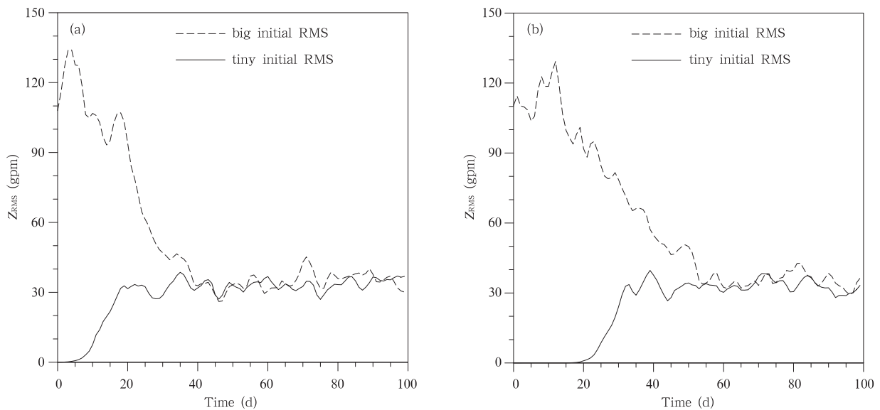
图 3 由 SAMIL 模拟得到的两组 REME 试验 500 hPa 位势高度场结果之间的均方根误差随时间的变化 (a. 单精度结果, b. 双精度结果; 虚线是每个初始场选 10 个样本做 REME 得到的结果, 第 1、2 组 REME 试验的初始场分别为第 30 年 1 月 1 日和第 31 年 1 月 1 日。实线是第 30 年 1 月 1 日的试验前 10 个样本 REME 试验和后 10 个样本 REME 试验结果之间的 RMS 差别)
